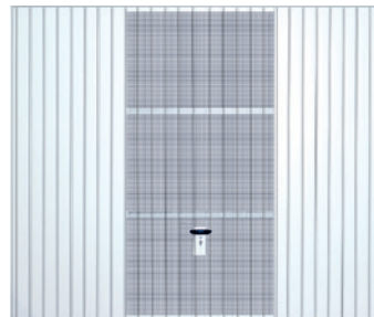
K 90 Typ Micro, 6 x 6 mm große Lüftungsöffnungen im Mittelblech
