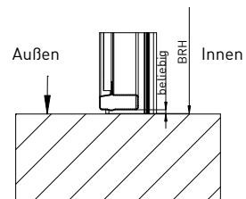
Außenanschlag durchgehender Boden Schwelle muss bauseits entfernt werden
