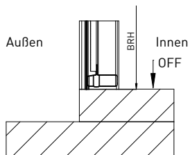
Innenanschlag Abkantung bauseits Schwelle muss bauseits entfernt werden
